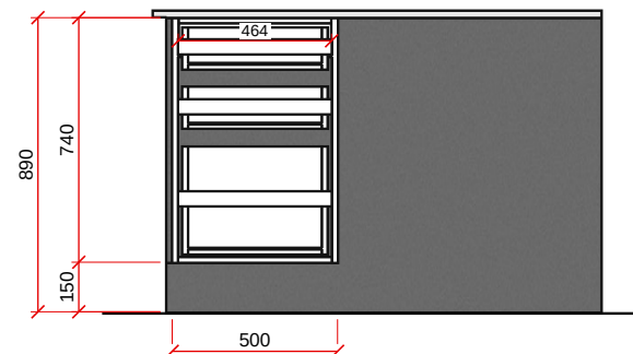
VISTA B - ESC. 1:25
