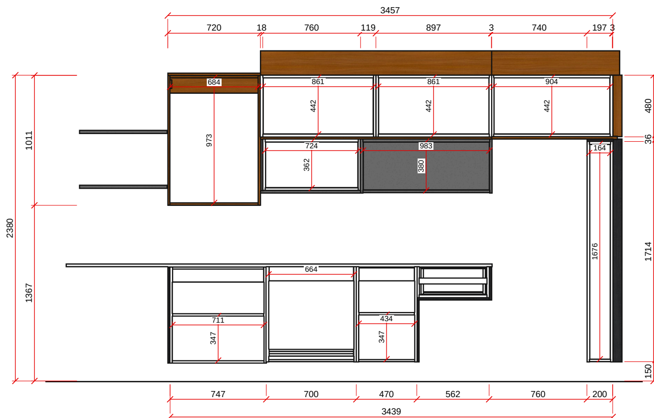
VISTA A - ESC. 1:30
